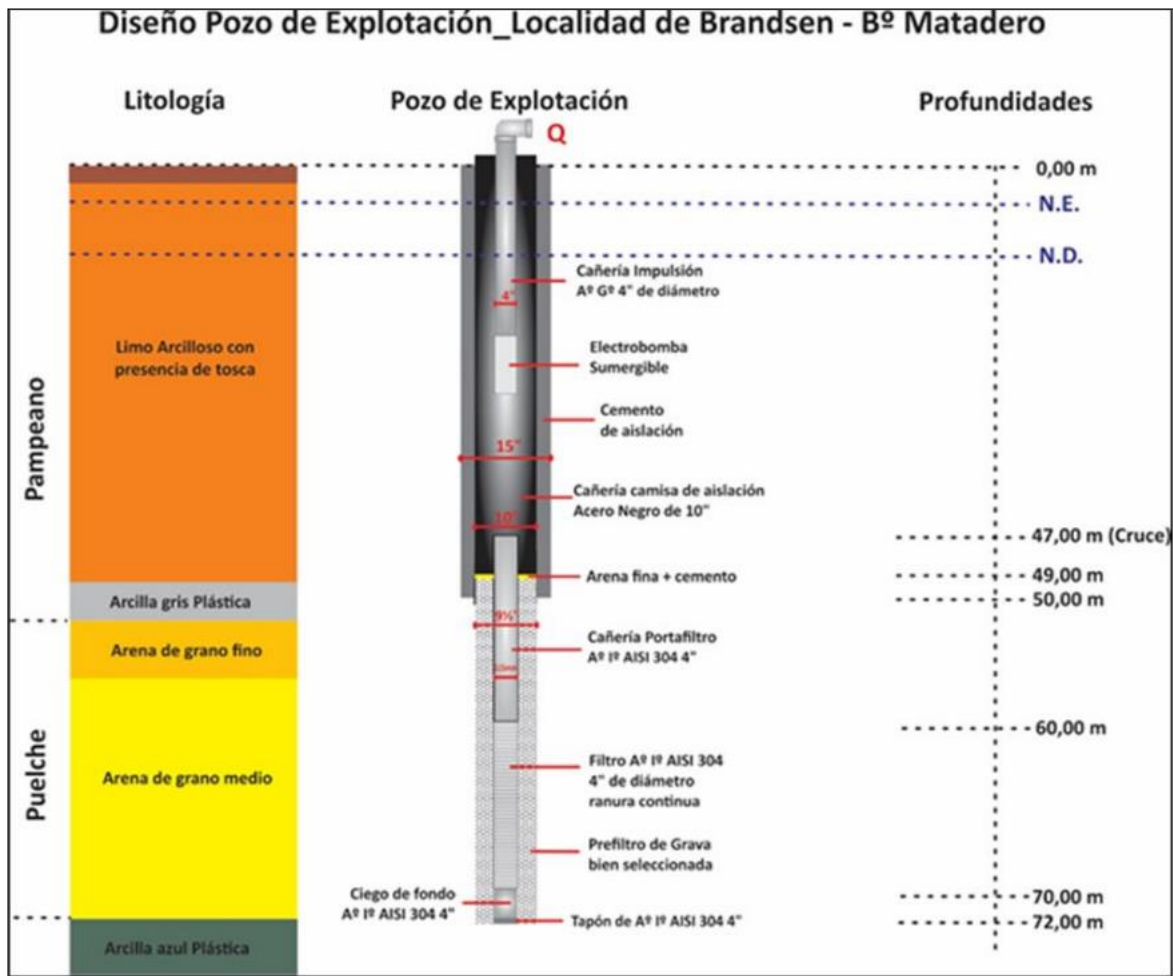
Figura 3: Esquema de los pozos de explotación
