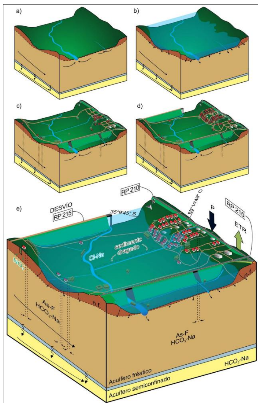
Figura 20: Modelo conceptual geohidrológico del río Samborombón en la localidad de Brandsen.
