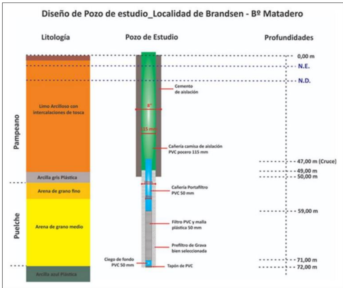
Figura 2: Esquema de perforaciones piloto.
