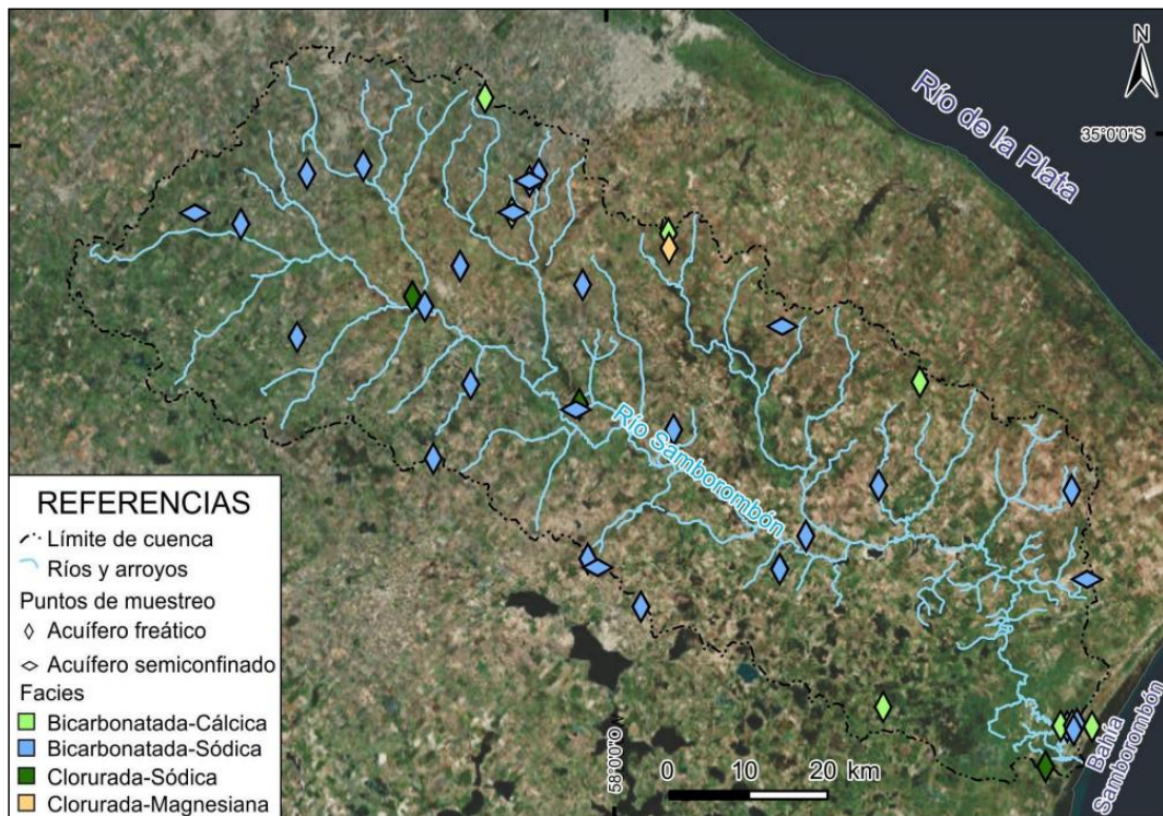
Figura 21: Distribución de facies del agua subterránea en la cuenca del río Samborombón.
