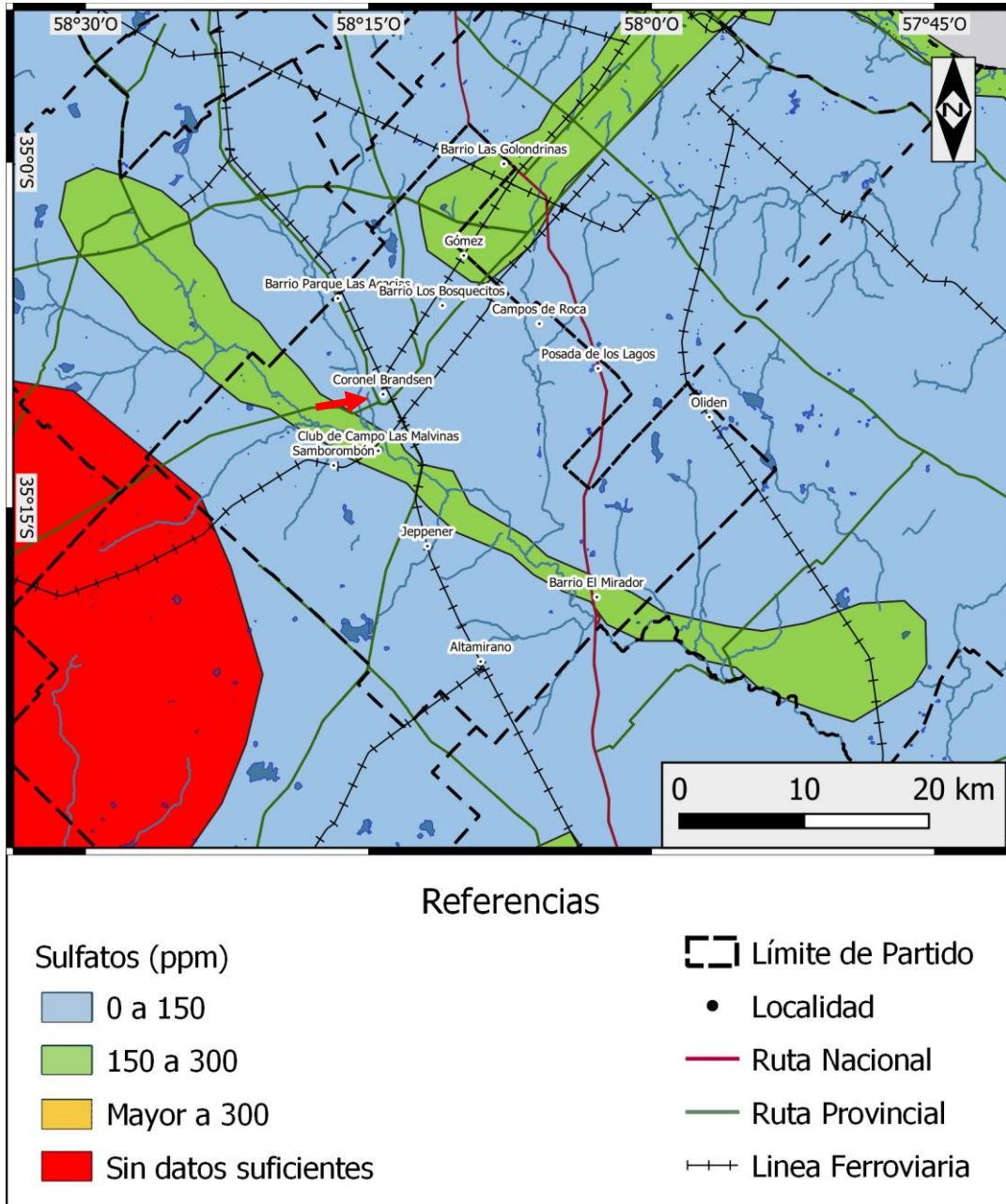
Figura 24: Mapa de concentración de sulfatos en el agua subterránea en el área de estudio (flecha) y su contexto próximo.
