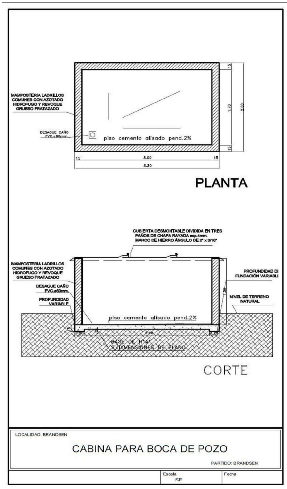
Figura 4: Esquema de cabina para boca de pozo.
