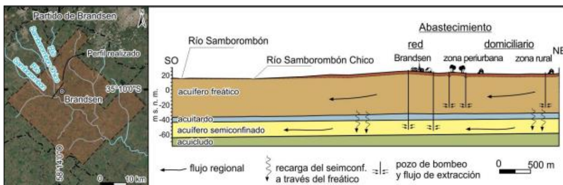
Figura 17: Perfil topográfico e hidrogeológico realizado en base a los registros de perforación en la localidad de Brandsen y alrededores. Las flechas negras indican la dirección del flujo tanto regional como local.
