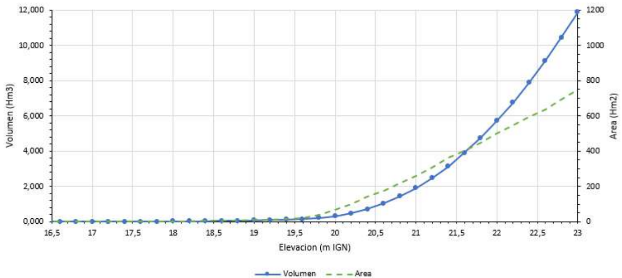
Figura 2-3. Curva de altura - volumen del Reservoirio R6.1.
