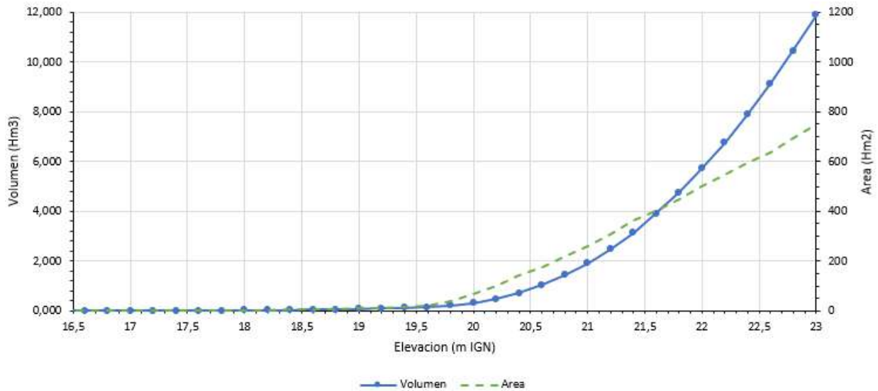
Figura 1-3. Curva de altura - volumen del Reservoirio R6.1.
