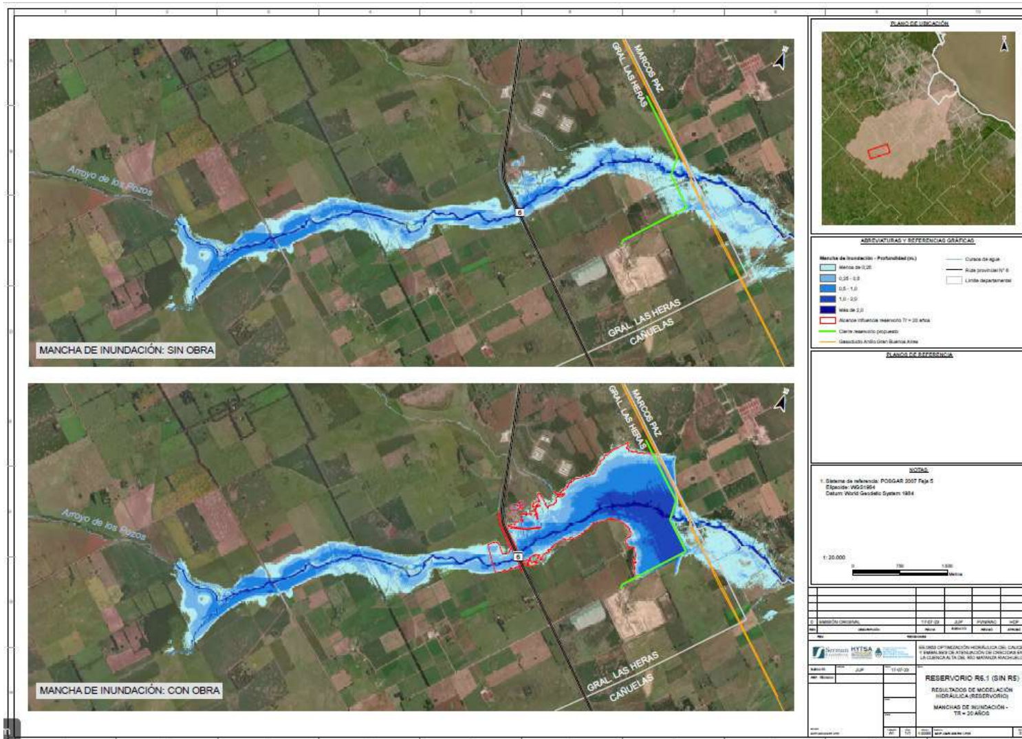
Figura 3-6. Manchas de inundación con una recurrencia de 20 años. Las tonalidades de azul denotan el nivel de agua: de más claro (menos profundo) a más oscuro (más profundo). En rojo se delimita el alcance de la influencia del reservorio.
