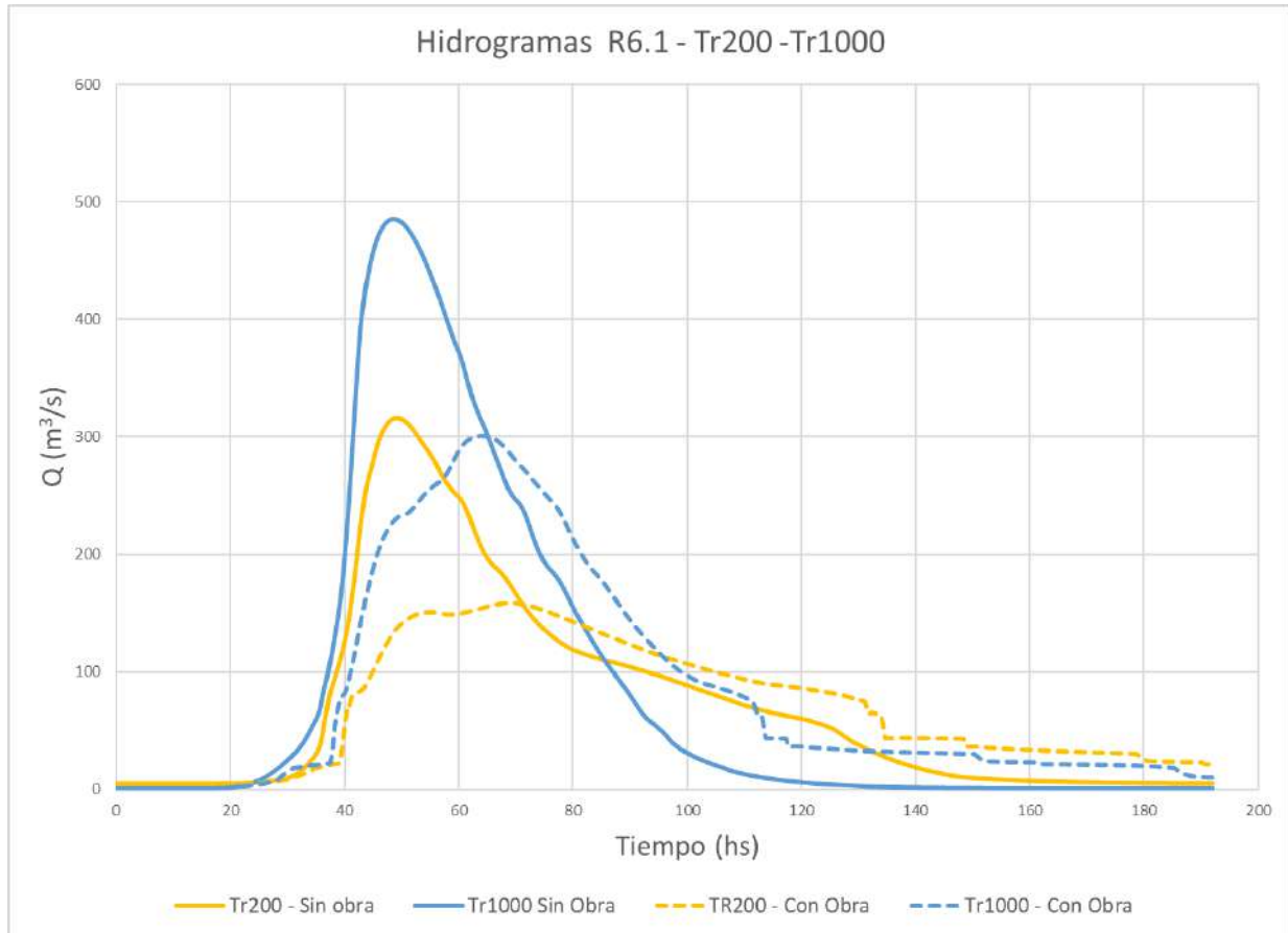
Figura 2-2. Atenuaciones generadas por el reservorio R6.1 para recurrencias de 200 y 1000 años.
