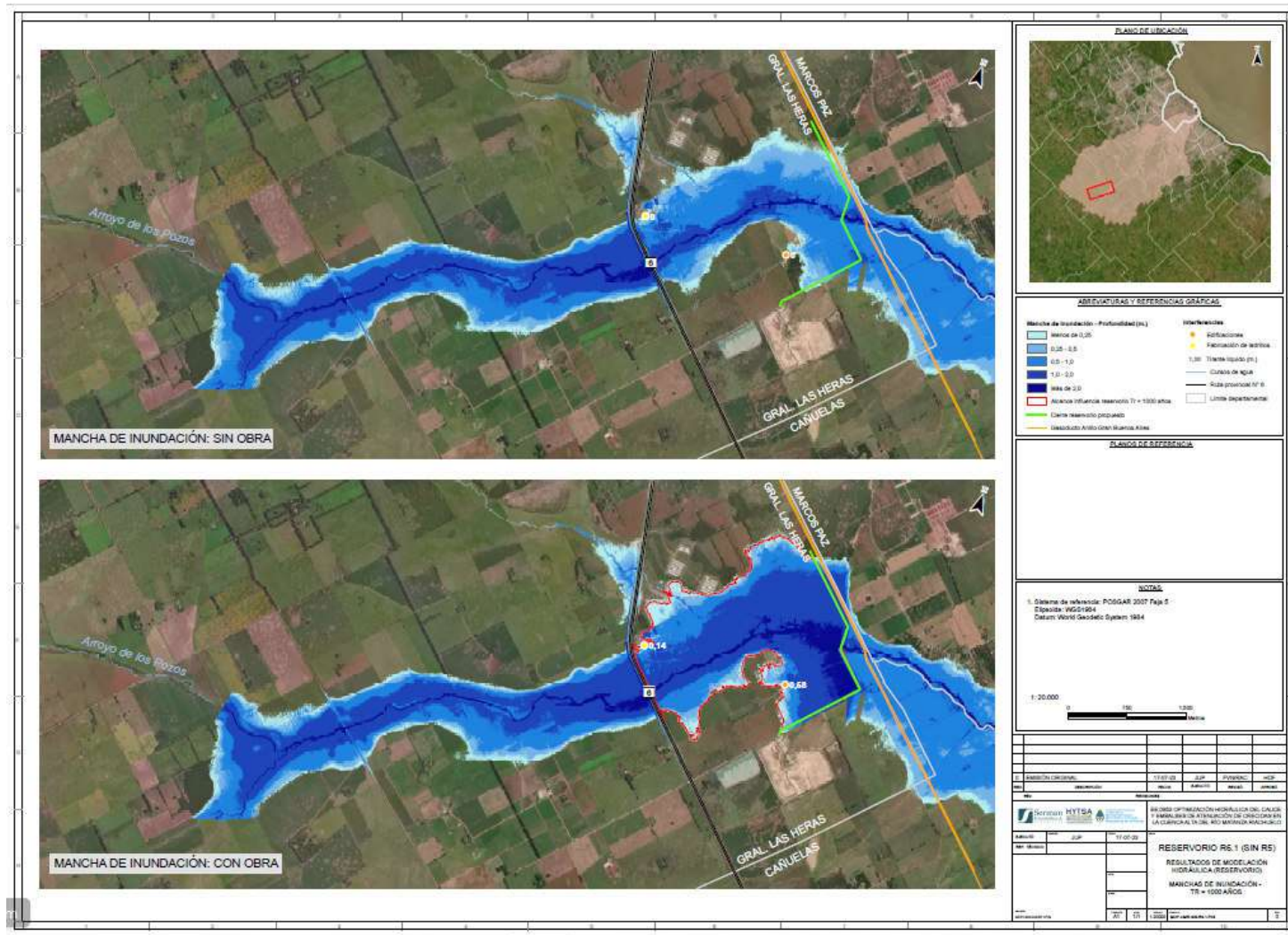
Figura 1-10. Manchas de inundación con una recurrencia de 1000 años. Las tonalidades de azul denota el nivel de agua: de más claro (menos profundo) a más oscuro (más profundo). En rojo se delimita el alcance de la influencia del reservorio.
