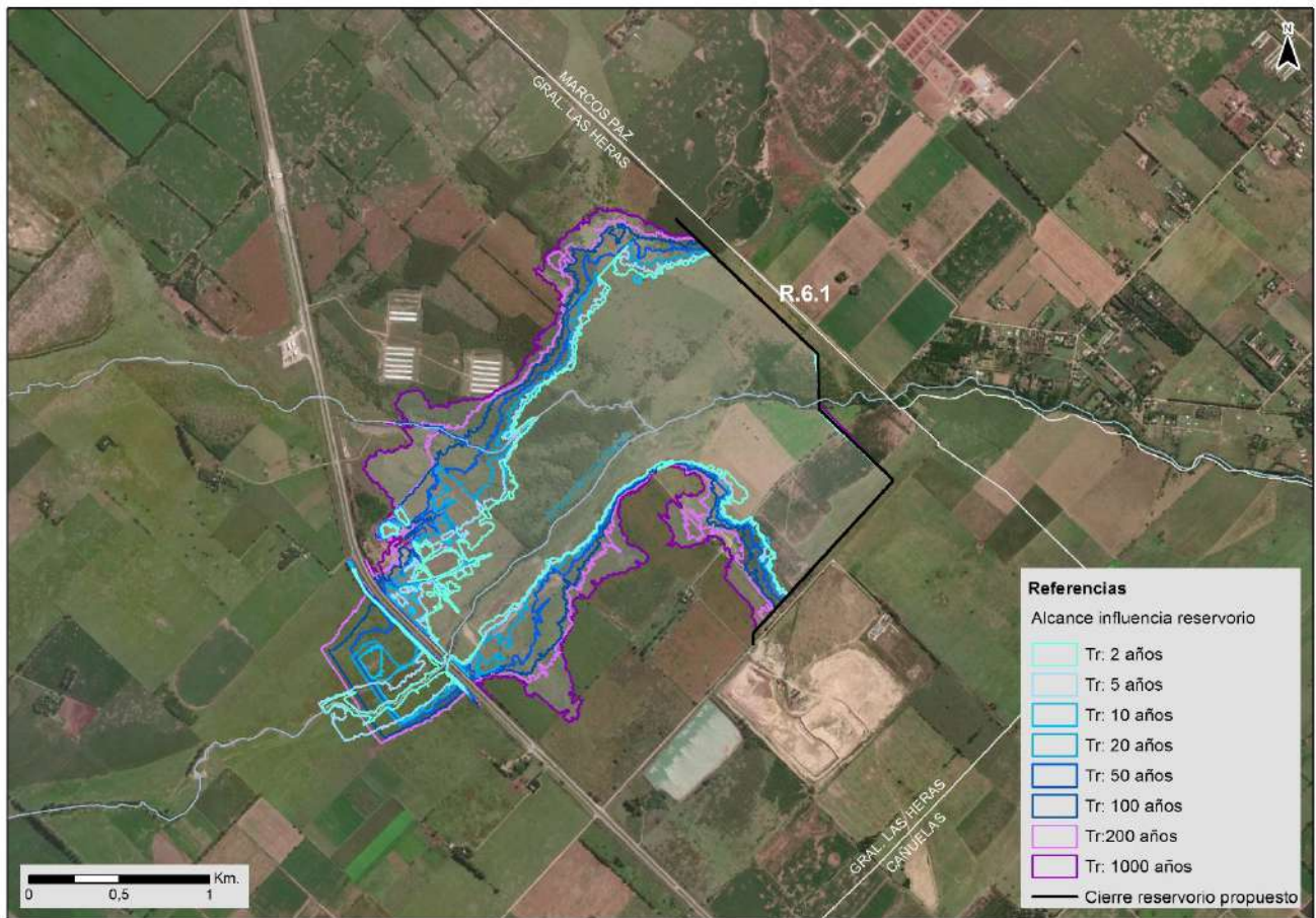
Figura 2-3. Influencia de reservorio para diferentes recurrencias.
