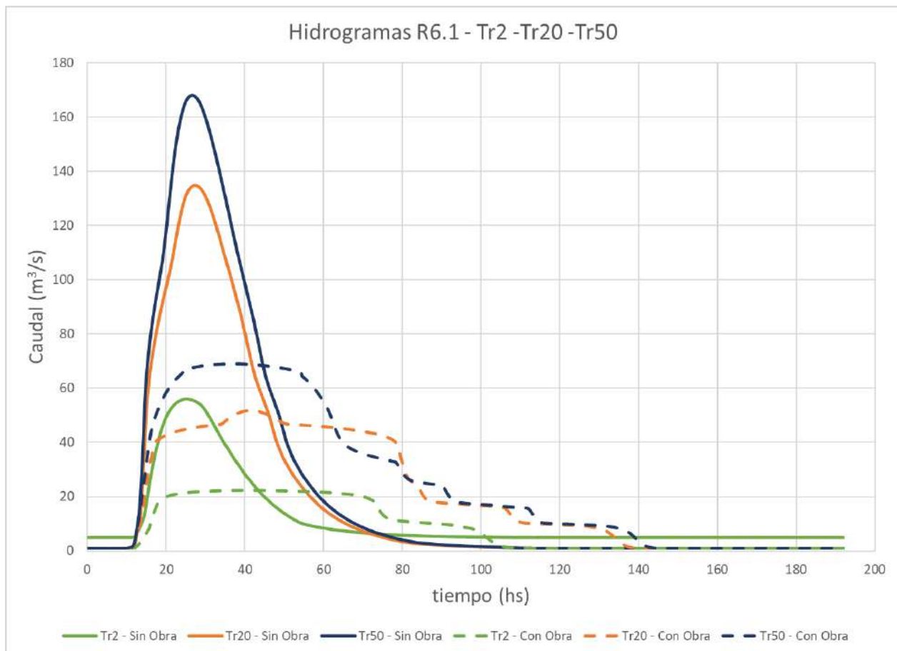
Figura 3-1. Hidrograma con obras y sin obras para las diferentes crecidas: 2, 20 y 50 años.
