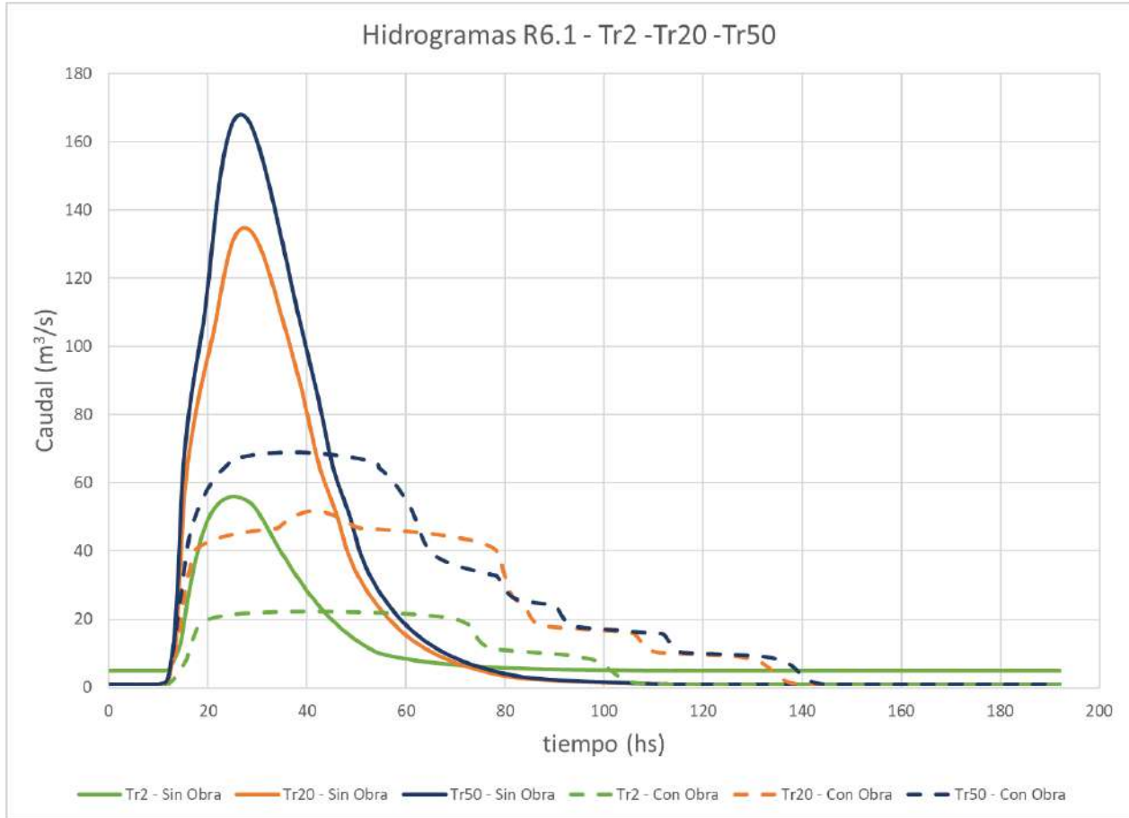
Figura 2-1. Atenuaciones generadas por el reservorio R6.1 para recurrencias de 2, 20 y 50 años.
