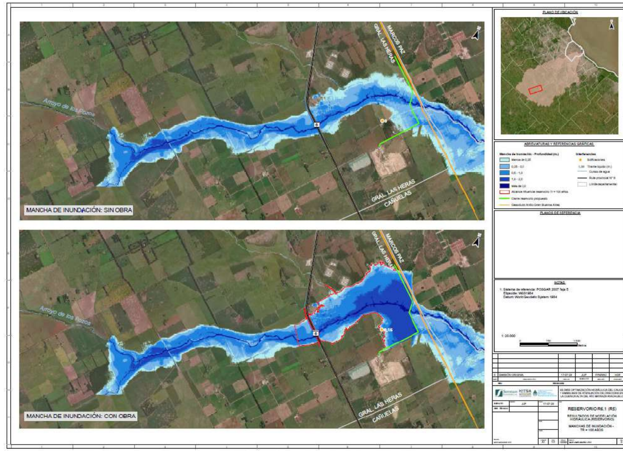
Figura 3-8. Manchas de inundación con una recurrencia de 100 años. Las tonalidades de azul denota el nivel de agua: de más claro (menos profundo) a más oscuro (más profundo). En rojo se delimita el alcance de la influencia del reservorio.
