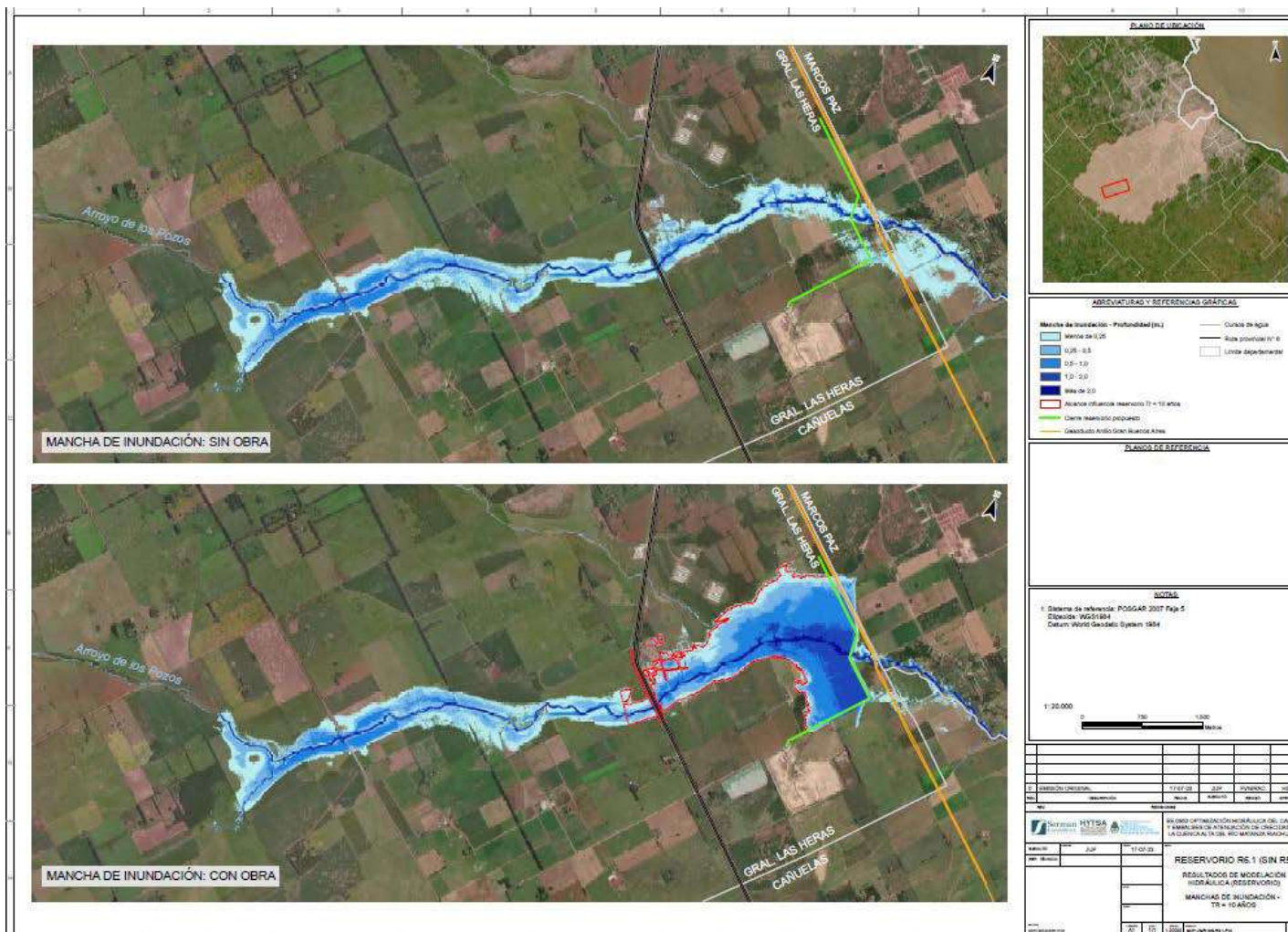
Figura 3-5. Manchas de inundación con una recurrencia de 10 años. Las tonalidades de azul denotan el nivel de agua: de más claro (menos profundo) a más oscuro (más profundo). En rojo se delimita el alcance de la influencia del reservorio.
