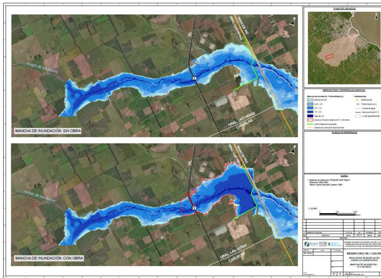
Figura 1-9. Manchas de inundación con una recurrencia de 200 años. Las tonalidades de azul denota el nivel de agua: de más claro (menos profundo) a más oscuro (más profundo). En rojo se delimita el alcance de la influencia del reservorio.
