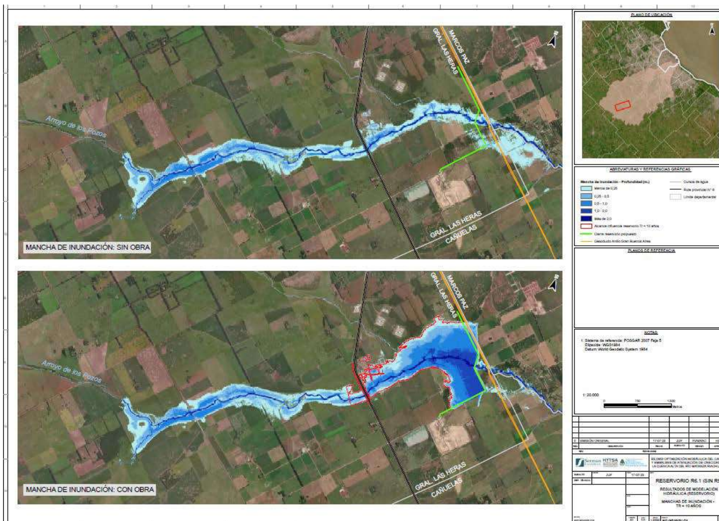
Figura 1-5. Manchas de inundación con una recurrencia de 10 años. Las tonalidades de azul denotan el nivel de agua: de más claro (menos profundo) a más oscuro (más profundo). En rojo se delimita el alcance de la influencia del reservorio.
