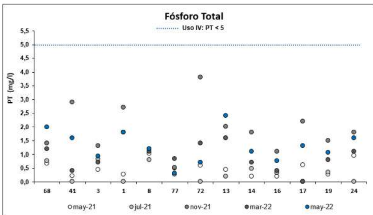
Figura 3-11. Evolución de Fósforo Total en cierres seleccionados de subcuencas. Fuente: CDCA ACUMAR.
