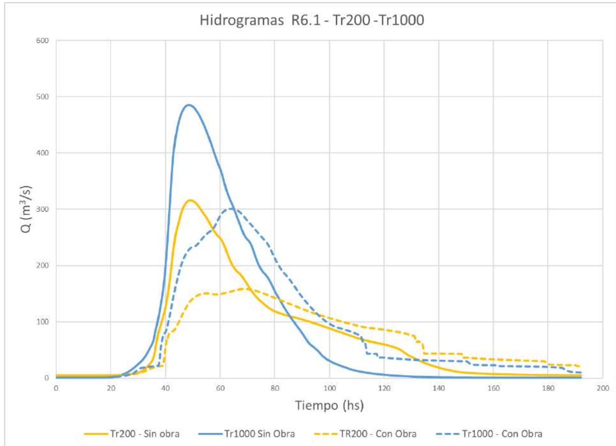
Figura 3-2. Atenuaciones generadas por el reservorio R6.1 para recurrencias de 200 y 1000 años.
