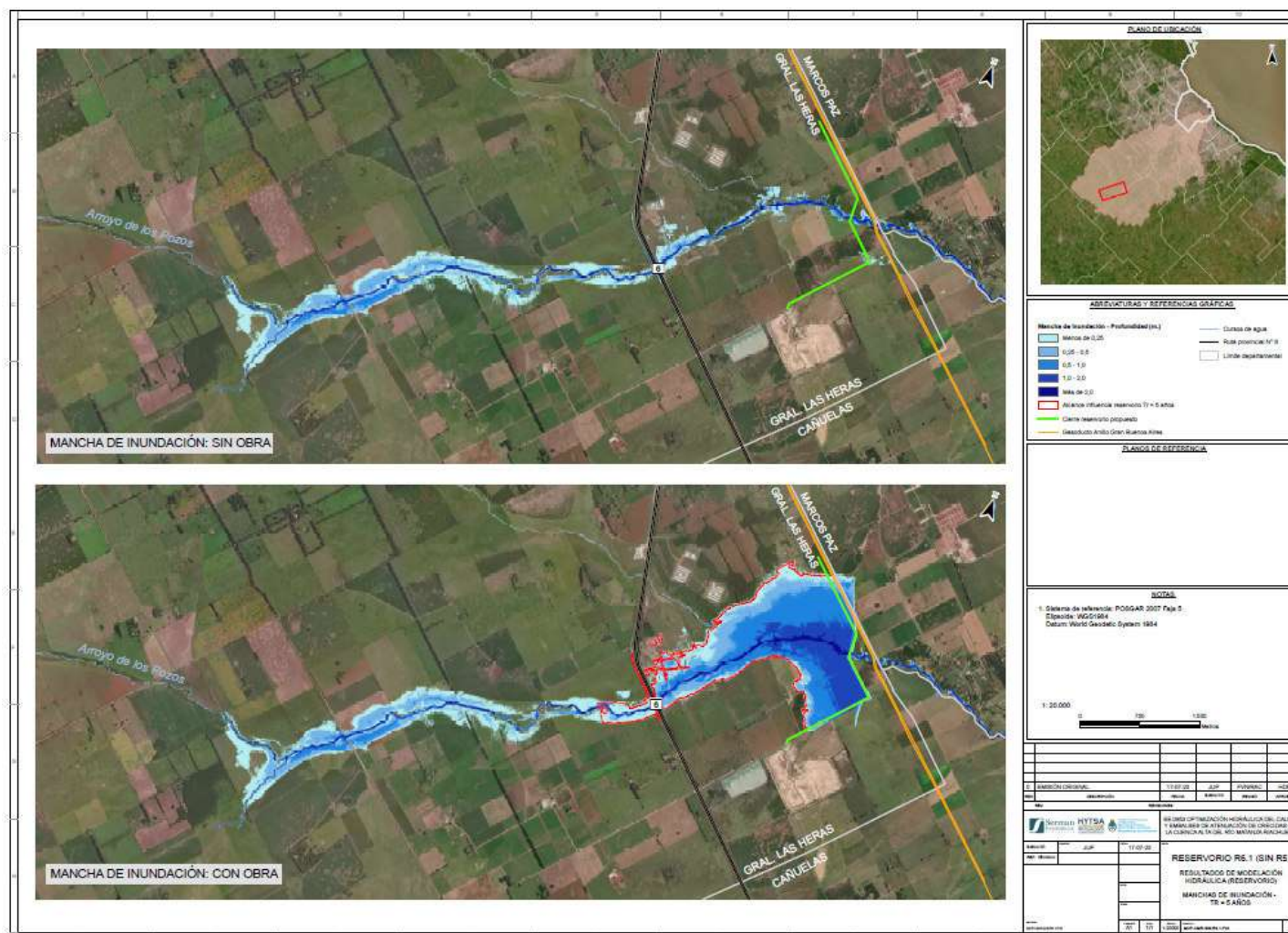
Figura 1-4. Manchas de inundación con una recurrencia de 5 años. Las tonalidades de azul denotan el nivel de agua: de más claro (menos profundo) a más oscuro (más profundo). En rojo se delimita el alcance de la influencia del reservorio.
