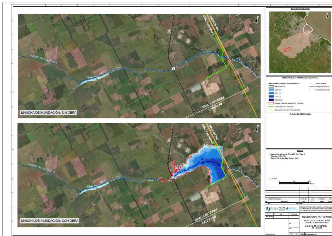
Figura 3-3. Manchas de inundación con una recurrencia de 2 años. Las tonalidades de azul denotan el nivel de agua: de más claro (menos profundo) a más oscuro (más profundo). En rojo se delimita el alcance de la influencia del reservorio.
