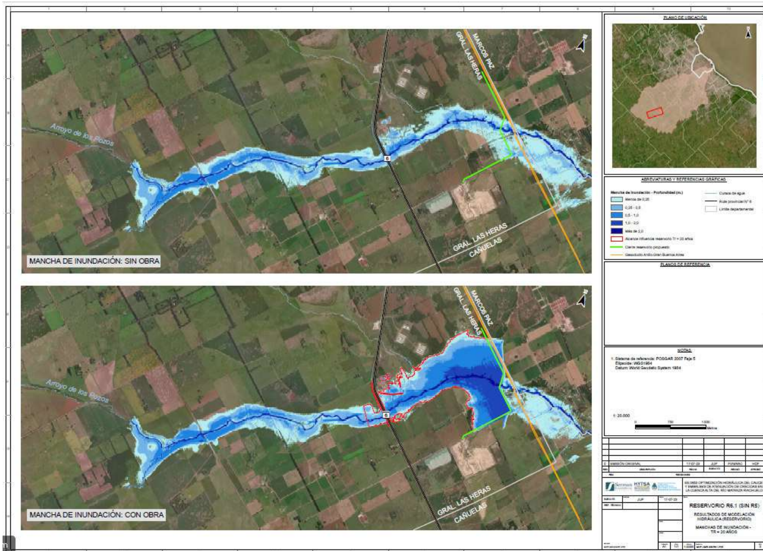
Figura 1-6. Manchas de inundación con una recurrencia de 20 años. Las tonalidades de azul denotan el nivel de agua: de más claro (menos profundo) a más oscuro (más profundo). En rojo se delimita el alcance de la influencia del reservorio.
