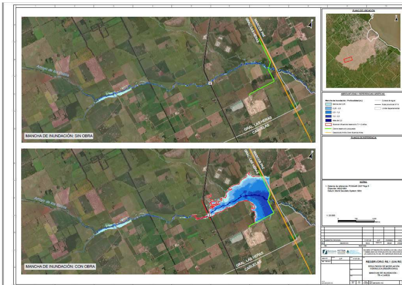
Figura 1-3. Manchas de inundación con una recurrencia de 2 años. Las tonalidades de azul denotan el nivel de agua: de más claro (menos profundo) a más oscuro (más profundo). En rojo se delimita el alcance de la influencia del reservorio.
