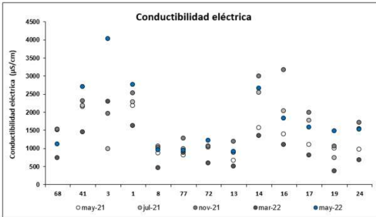
Figura 3-10. Evolución de conductividad eléctrica en cierres seleccionados de subcuencas. Fuente: CDCA ACUMAR
