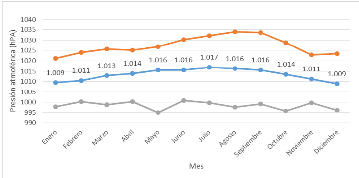
Figura 3-22. Presión atmosférica media mensual. Datos del Servicio Meteorológico Nacional. Estación meteorológica Ezeiza. Período 2011-2021.
