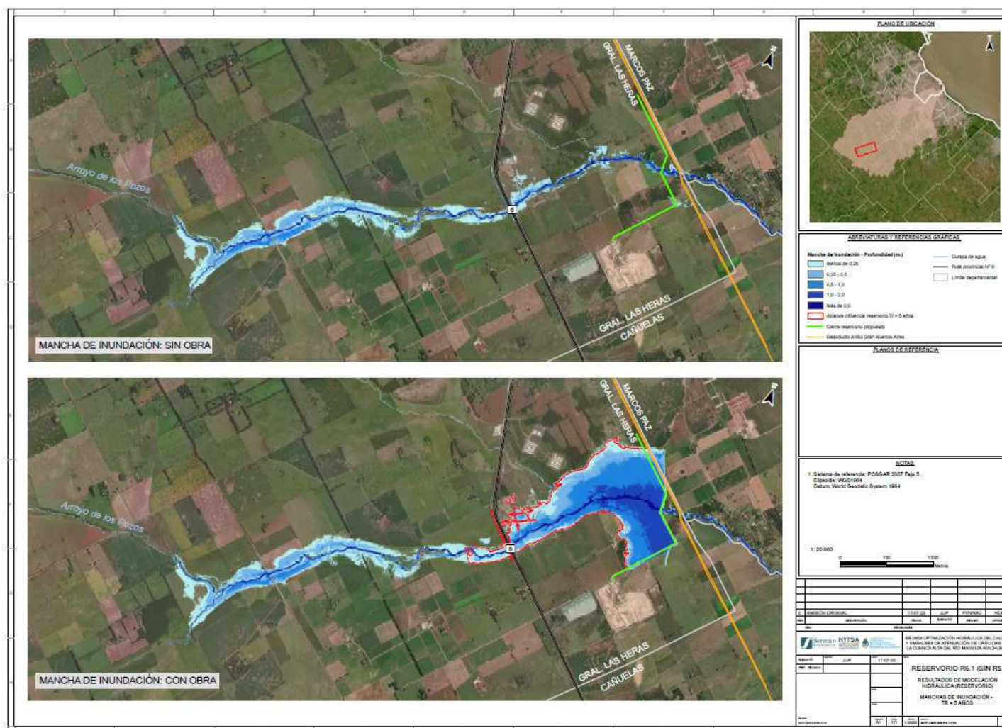
Figura 3-4. Manchas de inundación con una recurrencia de 5 años. Las tonalidades de azul denotan el nivel de agua: de más claro (menos profundo) a más oscuro (más profundo). En rojo se delimita el alcance de la influencia del reservorio.
