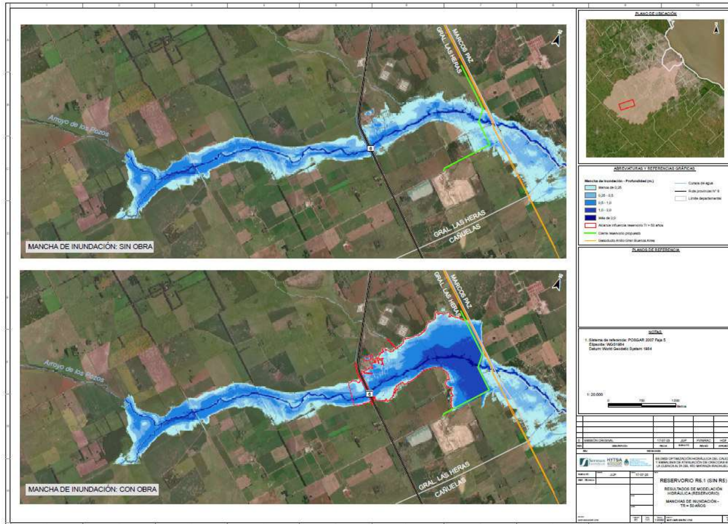
Figura 3-7. Manchas de inundación con una recurrencia de 50 años. Las tonalidades de azul denota el nivel de agua: de más claro (menos profundo) a más oscuro (más profundo). En rojo se delimita el alcance de la influencia del reservorio.
