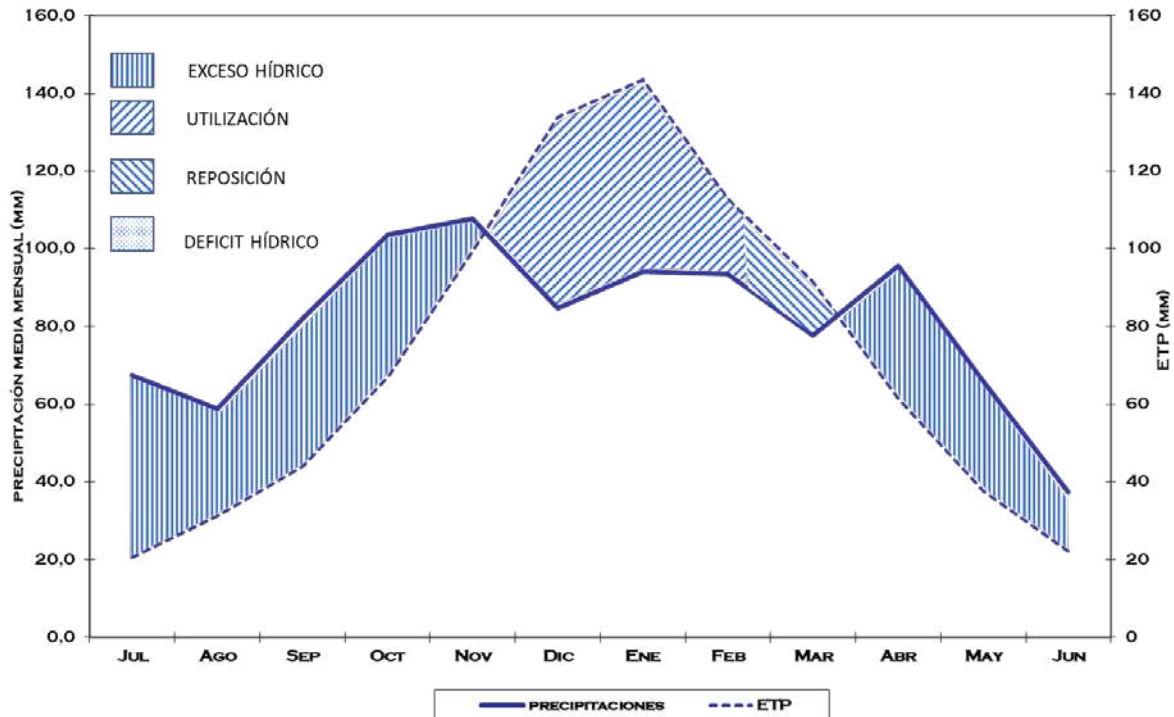
Figura 3-27. Balance hídrico para la estación meteorológica Ezeiza Aero. Datos del Servicio Meteorológico Nacional. Período 2011-2021.
