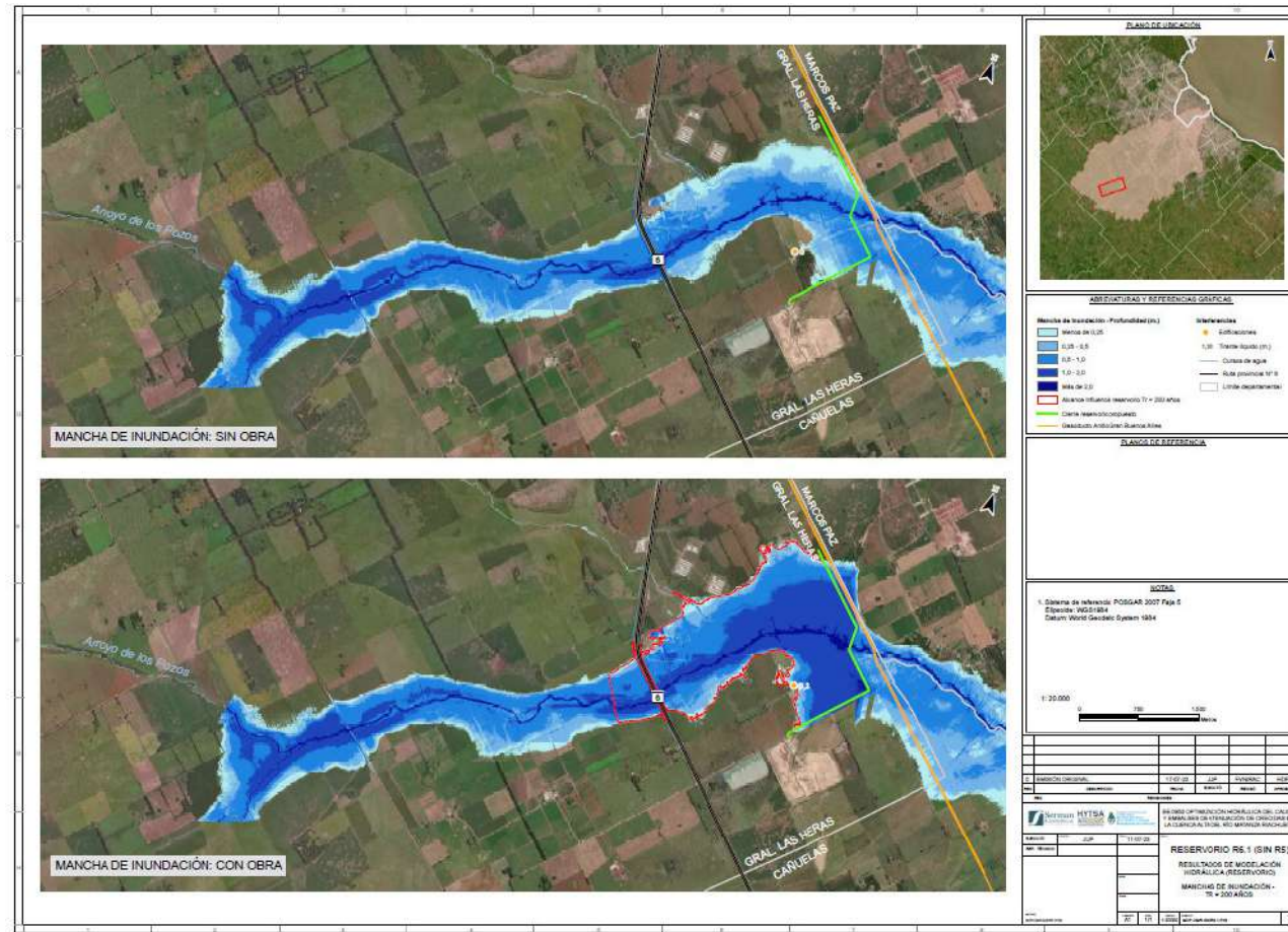
Figura 3-9. Manchas de inundación con una recurrencia de 200 años. Las tonalidades de azul denota el nivel de agua: de más claro (menos profundo) a más oscuro (más profundo). En rojo se delimita el alcance de la influencia del reservorio.
