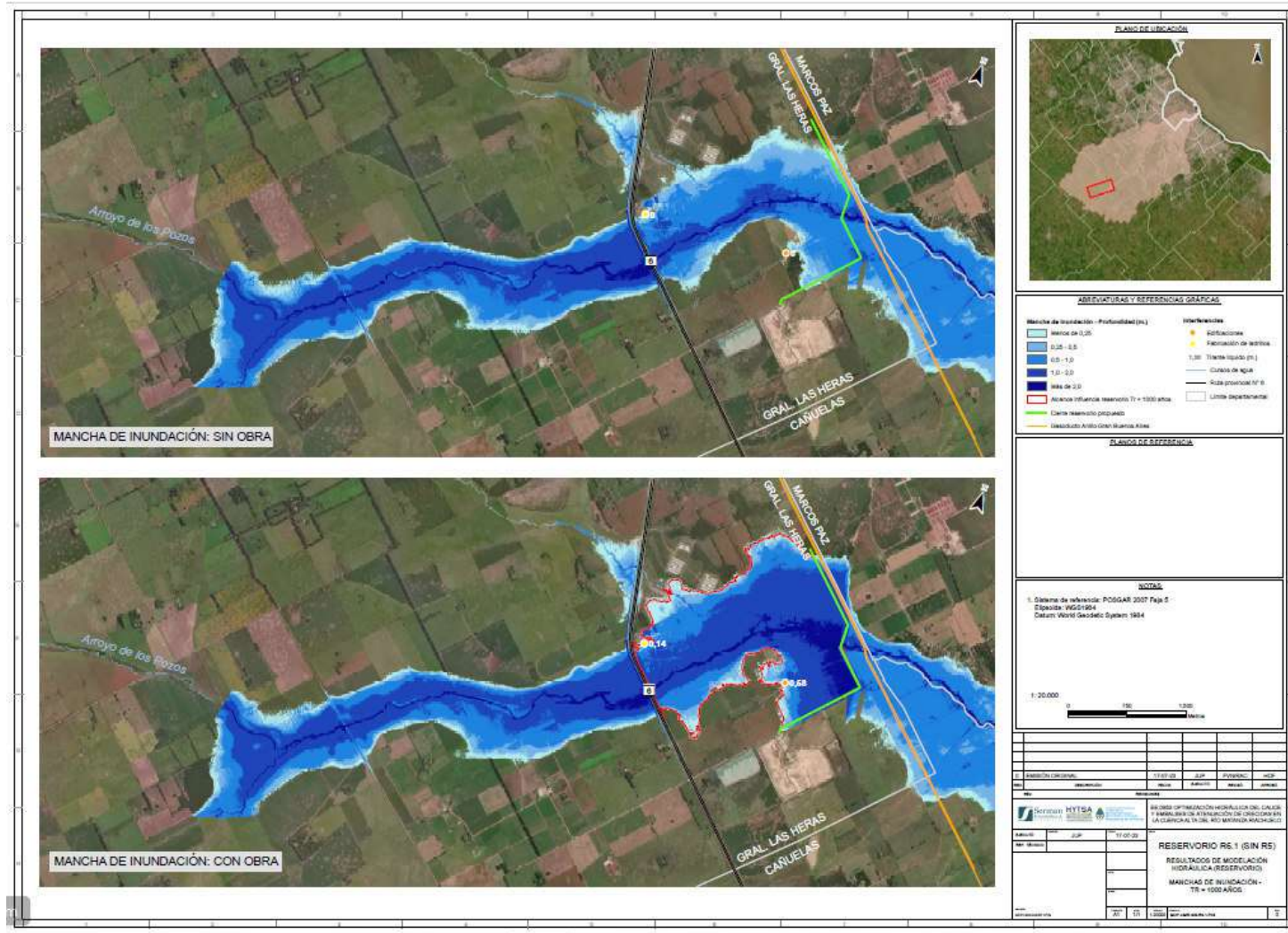
Figura 3-10. Manchas de inundación con una recurrencia de 1000 años. Las tonalidades de azul denota el nivel de agua: de más claro (menos profundo) a más oscuro (más profundo). En rojo se delimita el alcance de la influencia del reservorio.
