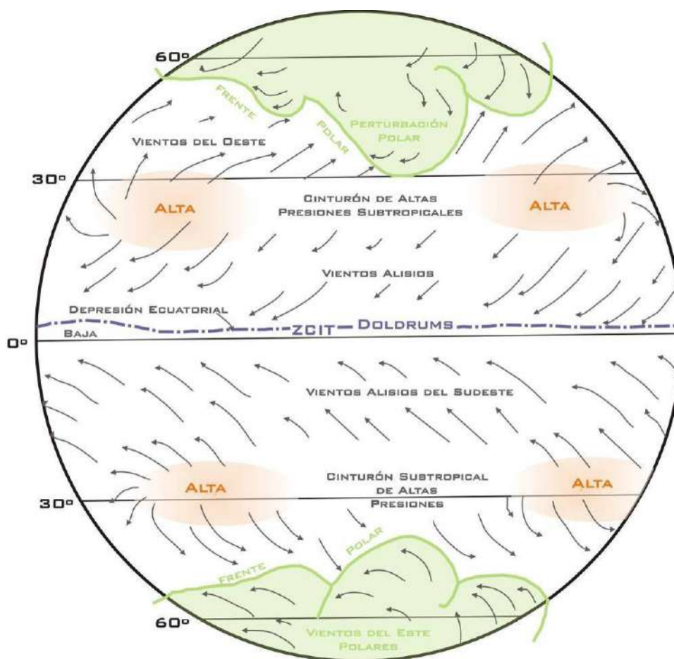
Figura 3-17. Esquema de los vientos planetarios en superficie (Strahler y Strahler, 2000).
