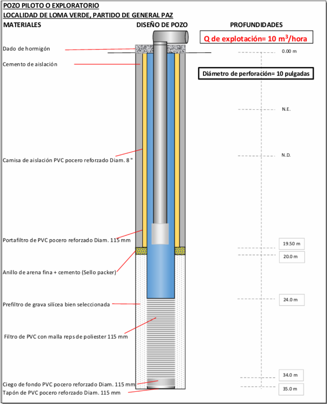
Figura 4: Esquema de perforaciones piloto.
