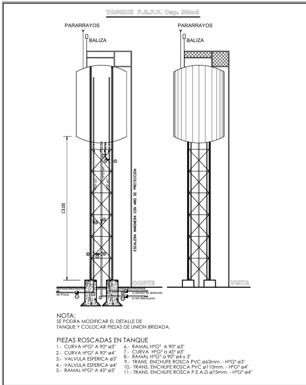
Figura 10: Plano tipo del Tanque de reserva.
