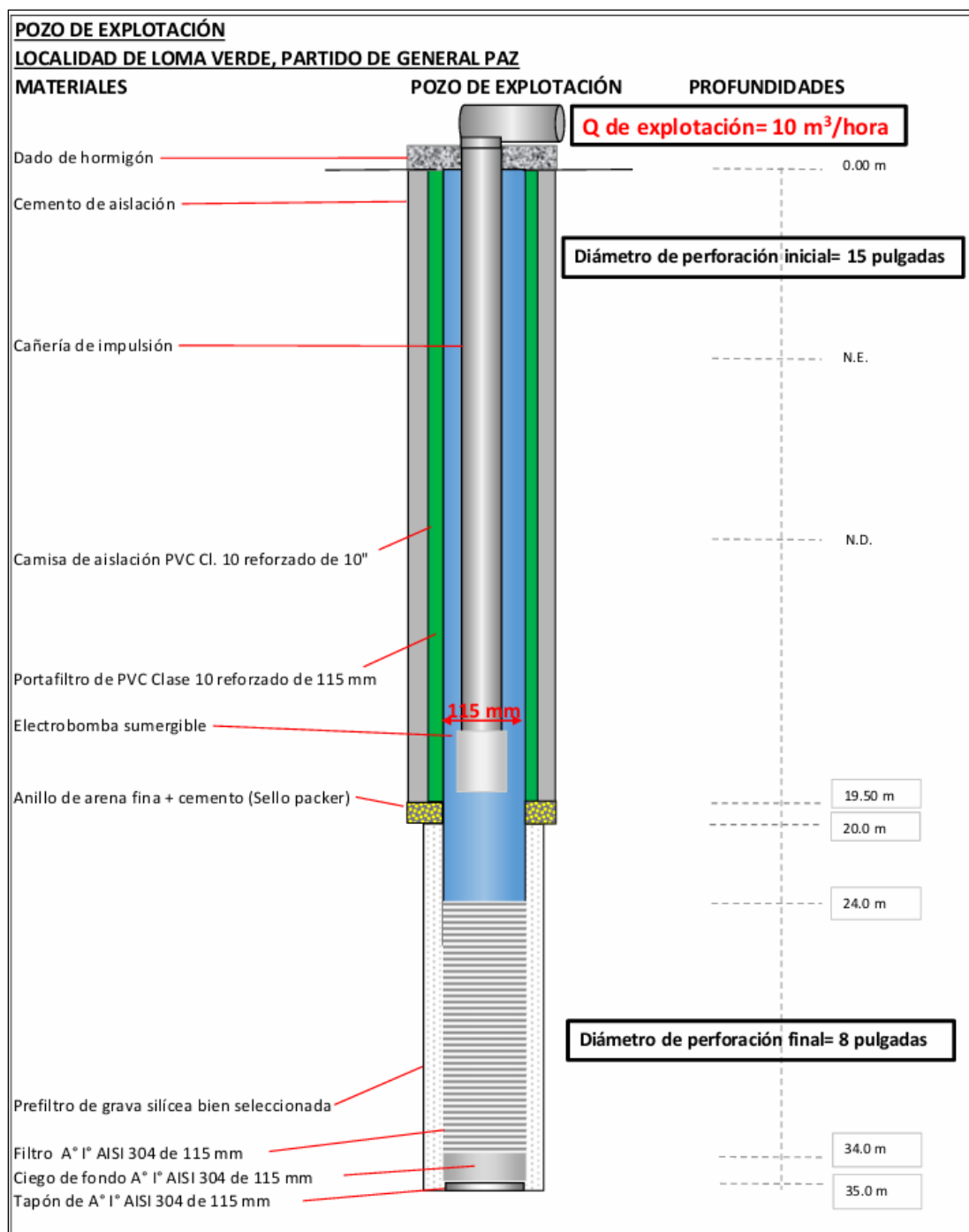
Figura 5: Esquema de los pozos de explotación
