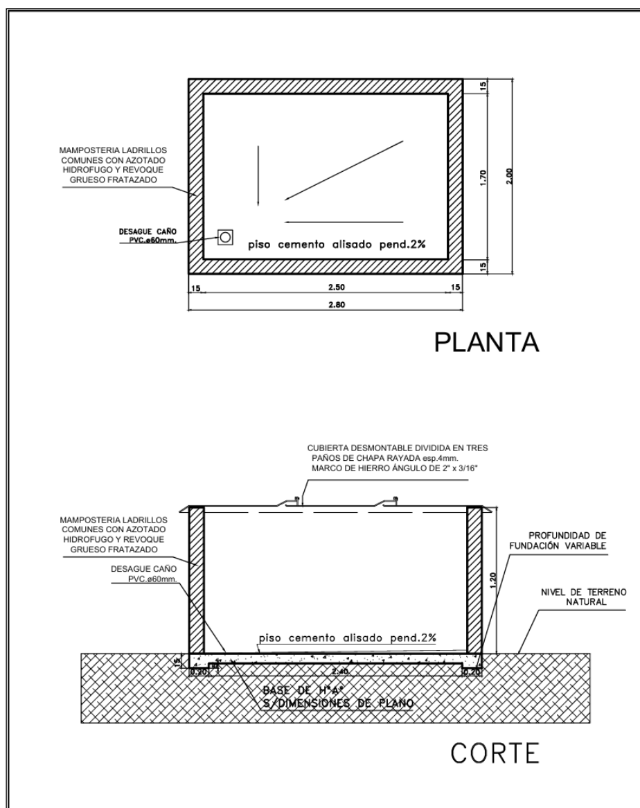
Figura 8: Cabina para boca de pozo.
