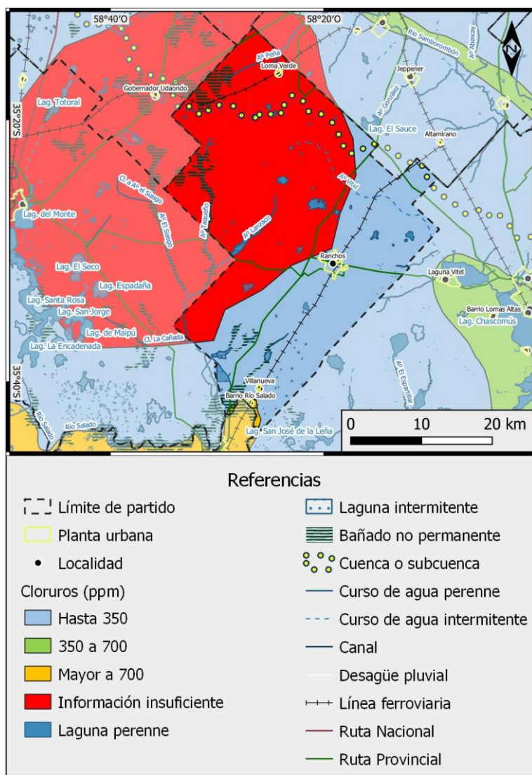
Figura 35: Mapa de salinidad del área de estudio y su contexto próximo.
