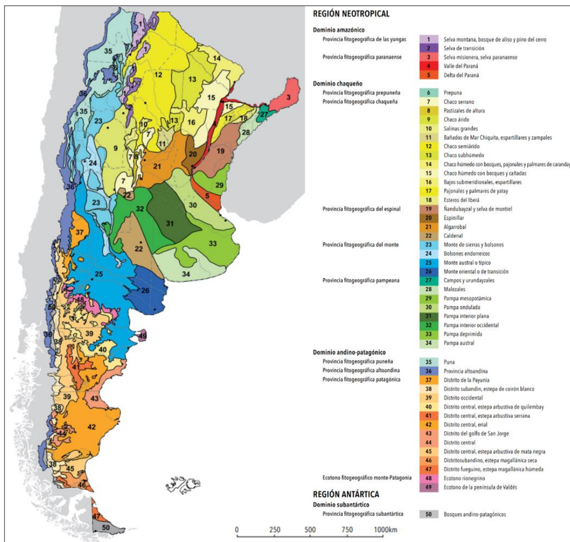
Figura 52: Mapa de unidades de vegetación de Argentina.
