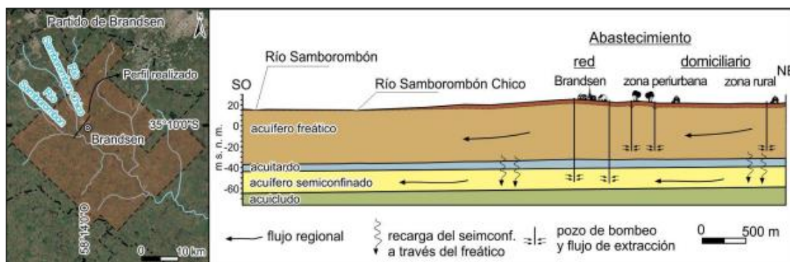
Figura 29: Perfil topográfico e hidrogeológico realizado en base a los registros de perforación en la localidad de Brandsen y alrededores.
