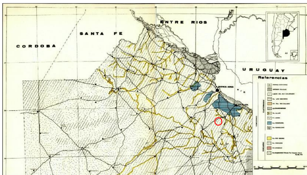
Figura 40: Mapa geológico parcial de la provincia de Buenos Aires. En el entorno del área estudiada (círculo rojo) se ubican las Fm. Buenos Aires, Luján y Junín.
