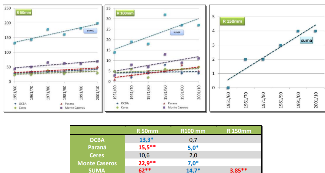
Figura 18: Aumento del número de casos de precipitaciones diarias que superan los umbrales (R) especificados, en periodos de 10 años.
