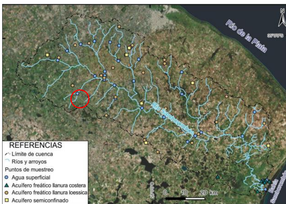
Figura 31: Ubicación de las muestras de agua analizadas por Borzi (2018).
