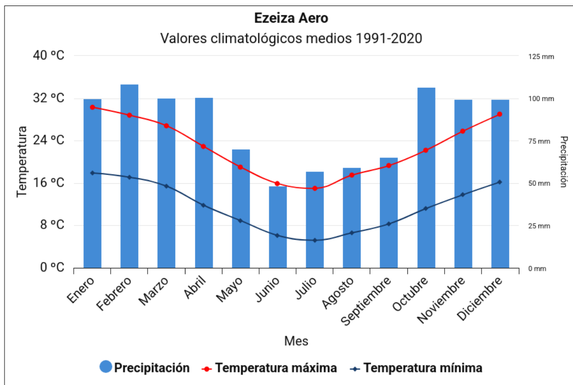
Figura 7: Valores medios mensuales de temperatura y precipitación en Ezeiza Aero.
