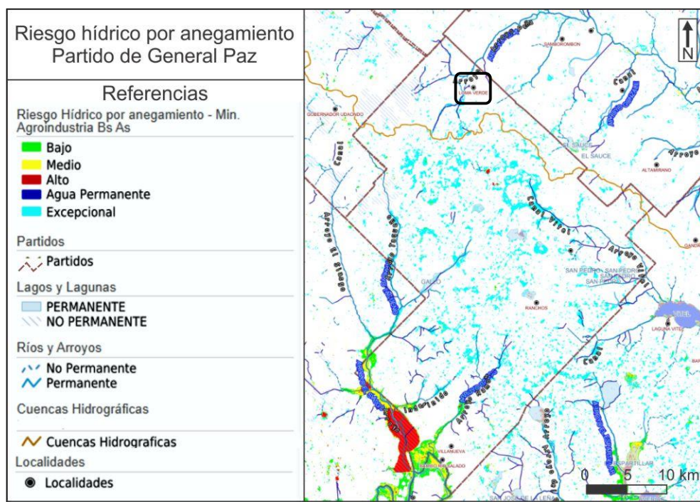
Figura 26: Riesgo hídrico en el Partido de General Paz. El recuadro negro indica la ubicación relativa del Proyecto.
