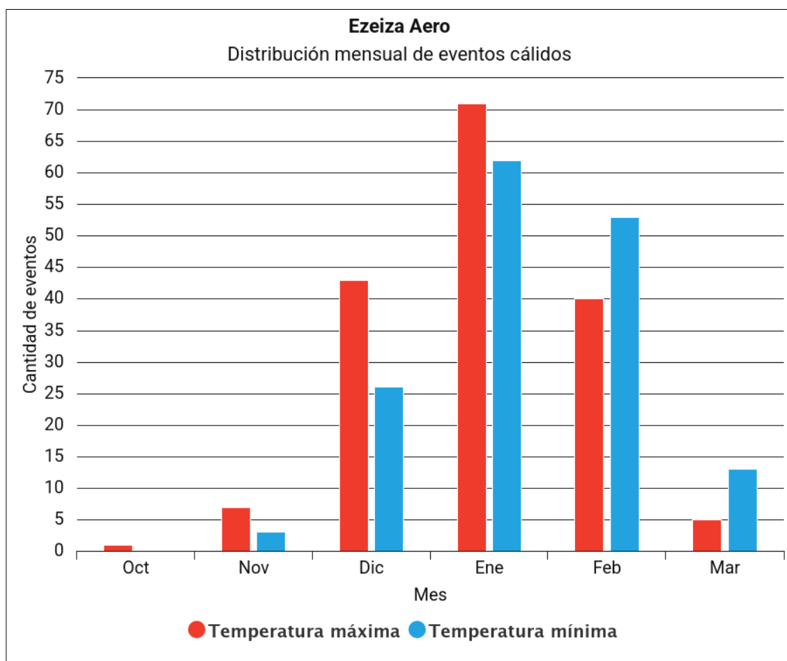
Figura 9: Cantidad de días con temperaturas extremas elevadas máximas (más de 32,5 °C) y mínimas (más de 20°C) en Ezeiza Aero.
