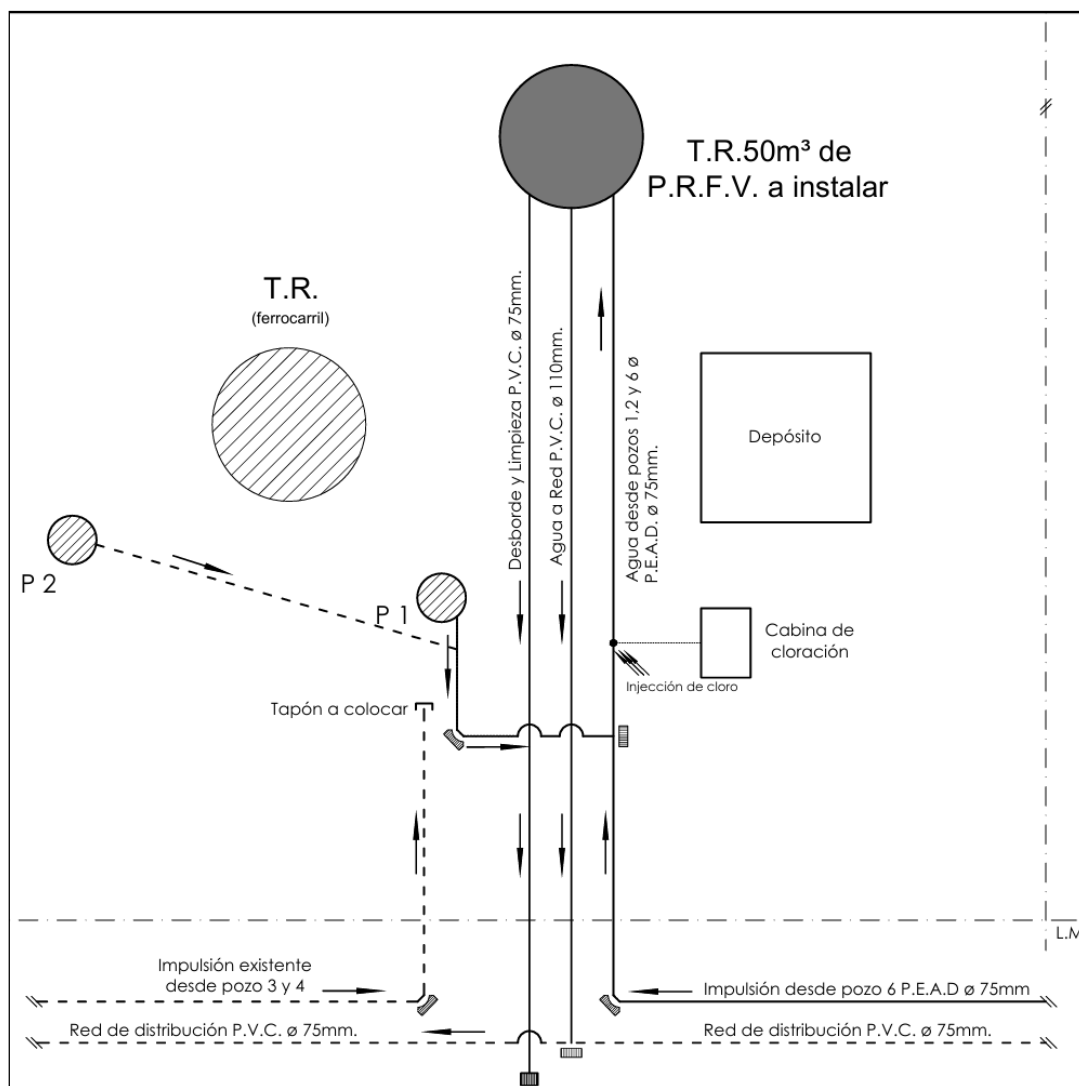
Figura 7: Detalle de las interconexiones en planta.
