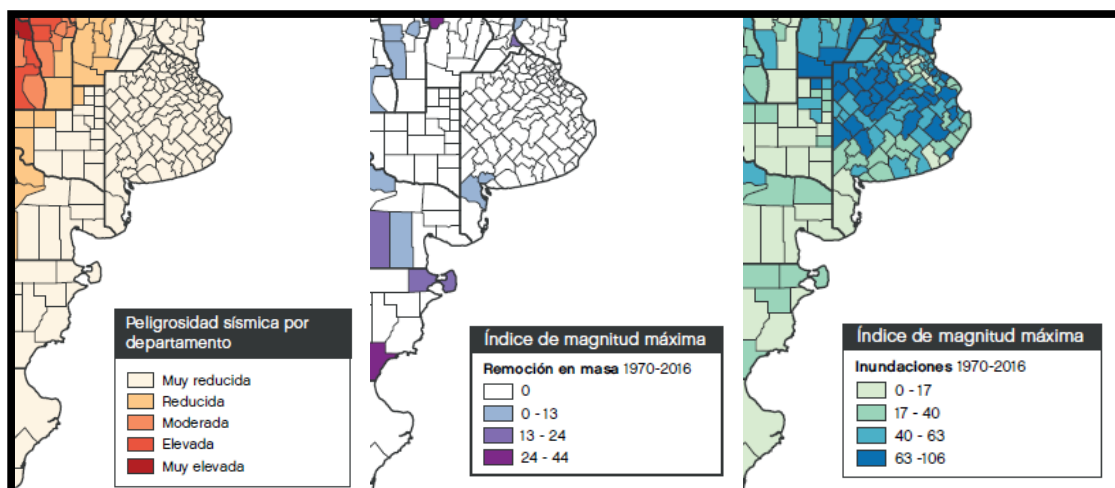
Figura 48: Característica de las diferentes amenazas: sísmica, remoción en masa e inundaciones.
