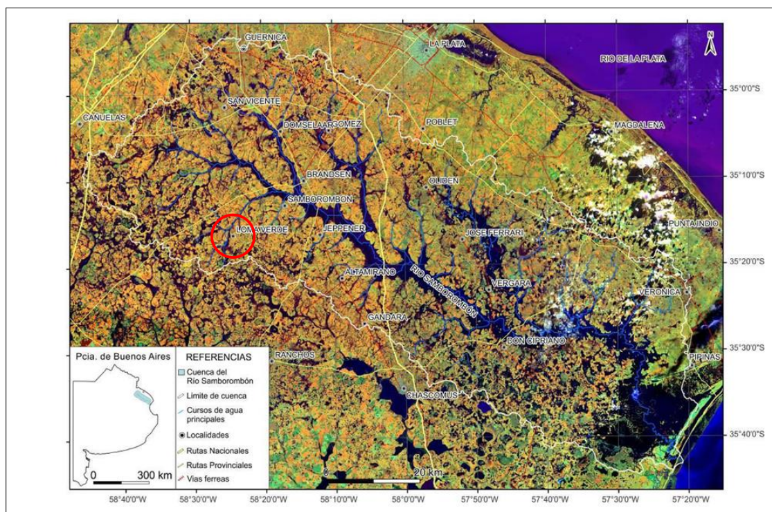
Figura 24: Ubicación de la cuenca del río Samborombón.
