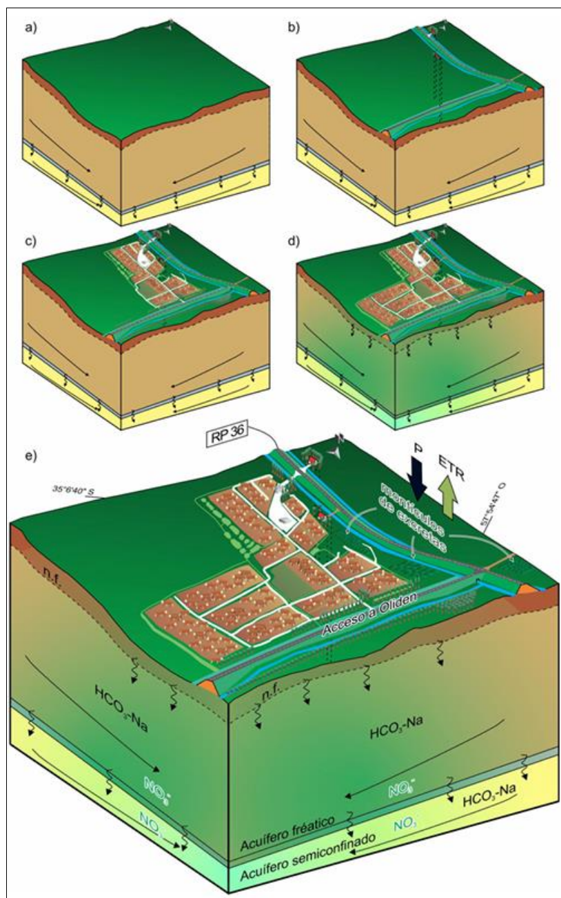
Figura 33: Modelo conceptual geohidrológico del río Samborombón en la localidad de Oliden.
