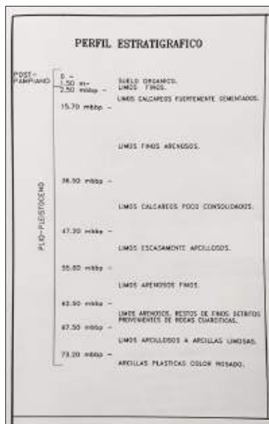
Figura 26: Perfil litológico de perforación del servicio de agua de Chasicó (1999).
