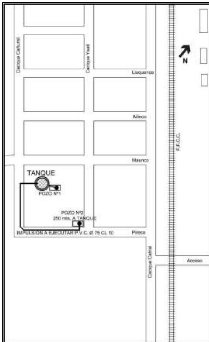
Figura 6: Ubicación de cañería de impulsión y pozos de explotación existente y a ejecutar.
