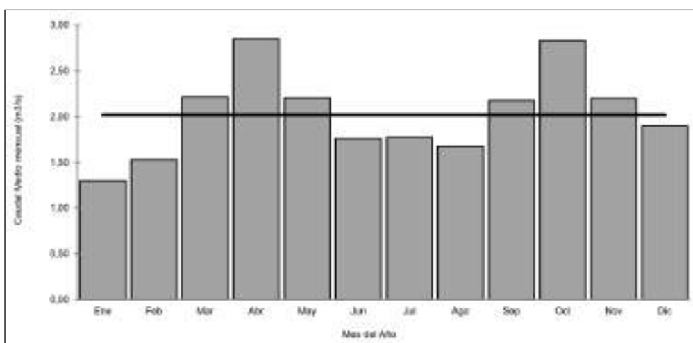
Figura 11: Río Sauce Chico – Estación HL6005 - Caudales Medios Mensuales (m 3 /s) y su comparación con el módulo anual.
