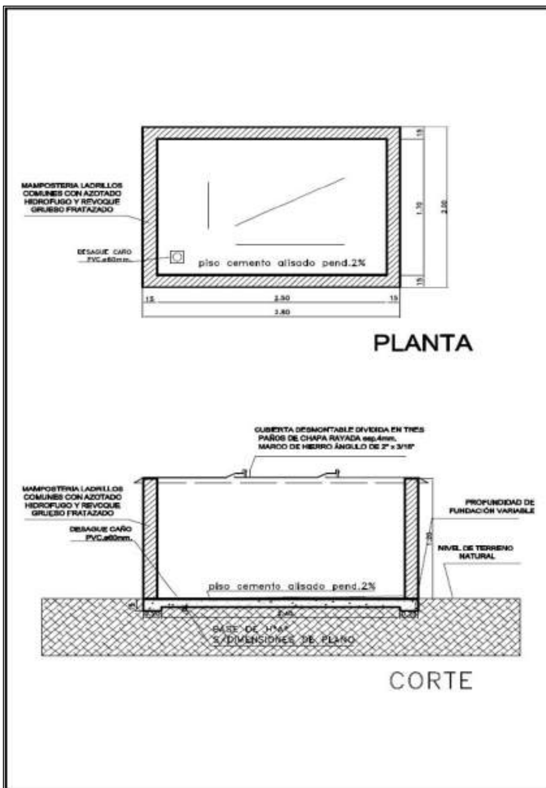
Figura 8: Esquema de cabina para boca de pozo.
