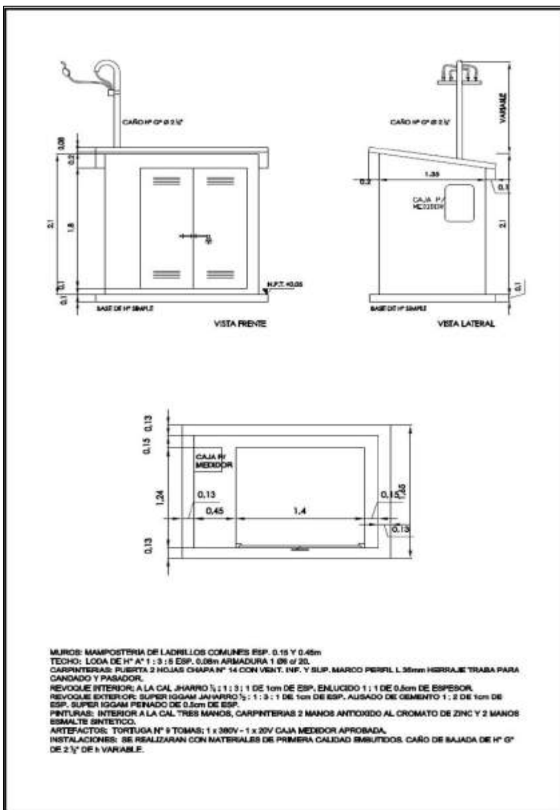
Figura 7: Esquema de cabina para tablero.
