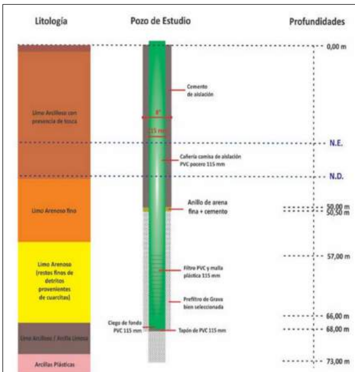
Figura 3: Esquema del pozo exploratorio
