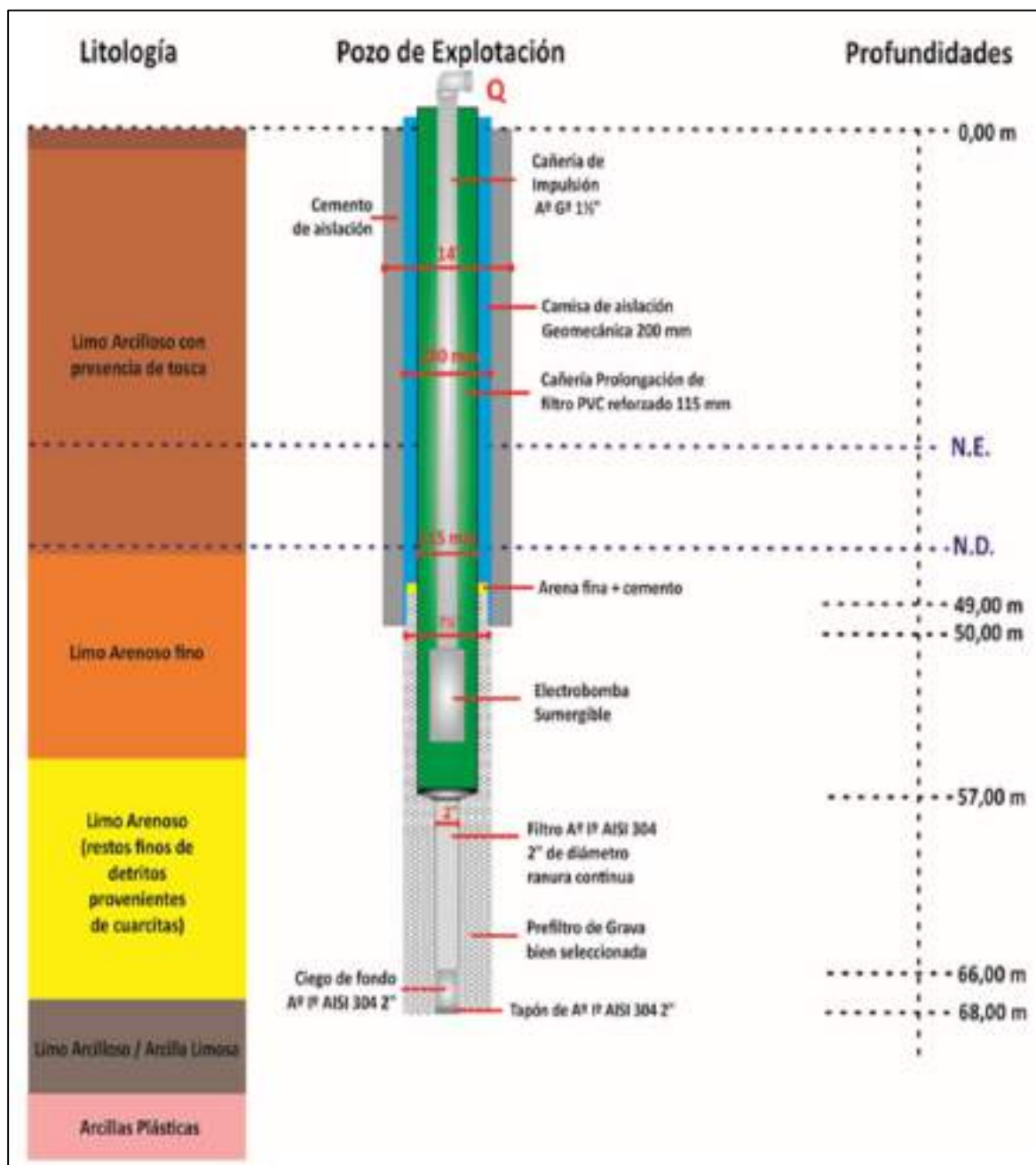
Figura 4: Esquema pozo de explotación
