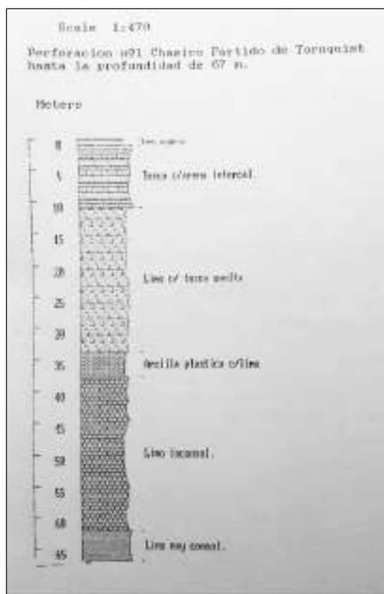
Figura 25: Perfil litológico de perforación de estudio en Chasicó (1992).
