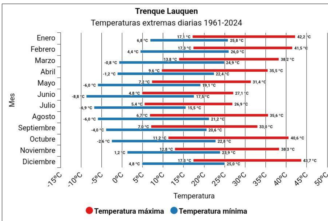
Figura 9: Cantidad de días con temperaturas extremas elevadas máximas y mínimas en Trenque Lauquen.
