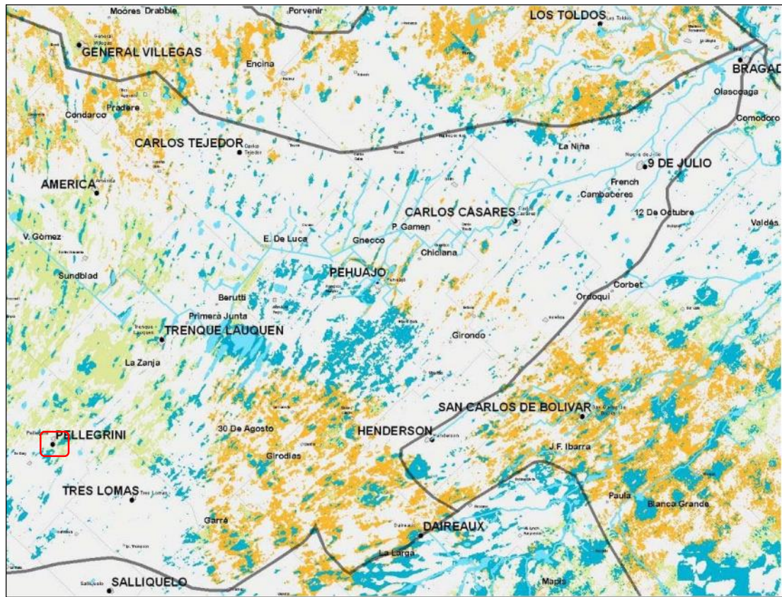
Figura 34: Mapa de inundaciones modeladas para 2 (azul), 5 (verde) y 10 (anaranjado) años de recurrencia incorporando las obras propuestas. El recuadro rojo indica la ubicación del Proyecto.
