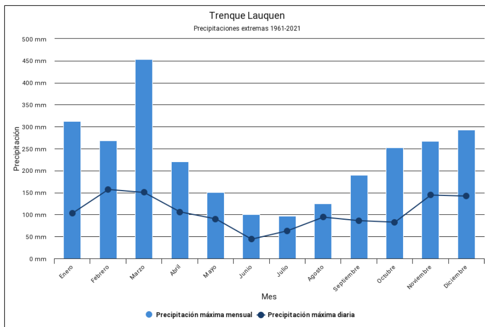
Figura 8: Precipitaciones extremas mensuales (barras) y diarias (puntos) en Trenque Lauquen.
