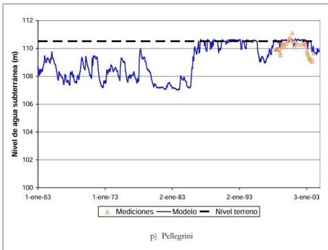
Figura 35: Variación modelada del nivel freático y mediciones en la localidad de Pellegrini.
