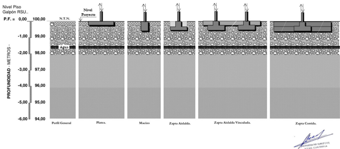
Fig. Esquema de las fundaciones. Fuente: Estudio de suelo del proyecto.
