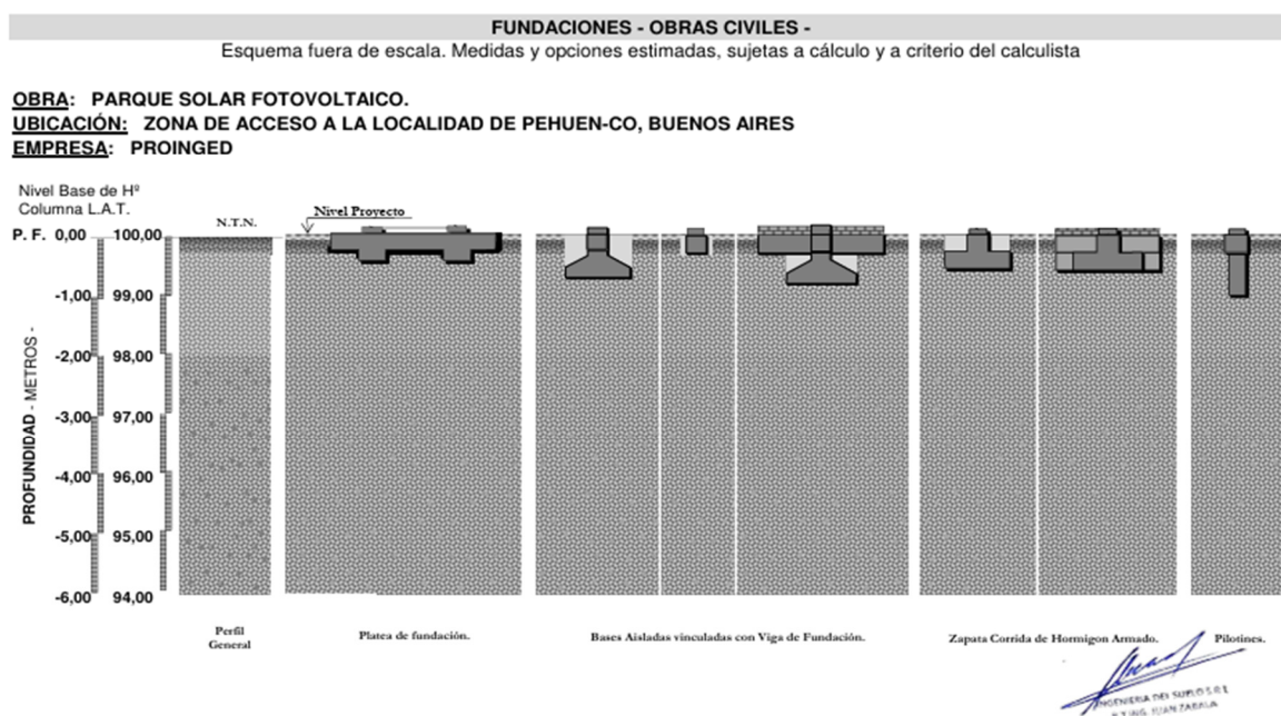
Fig. Esquema de las fundaciones. Fuente: Estudio de suelo del proyecto.
